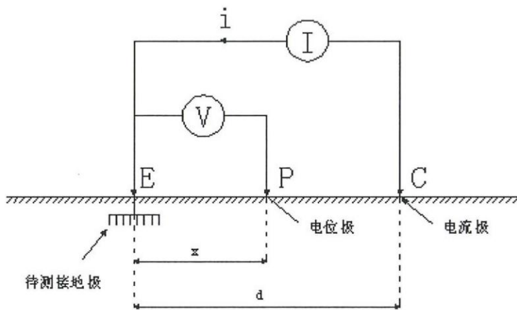
图B.1 接线原理图
