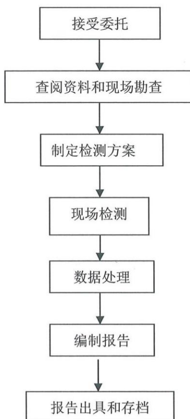
图1 防雷装置检测流程图
