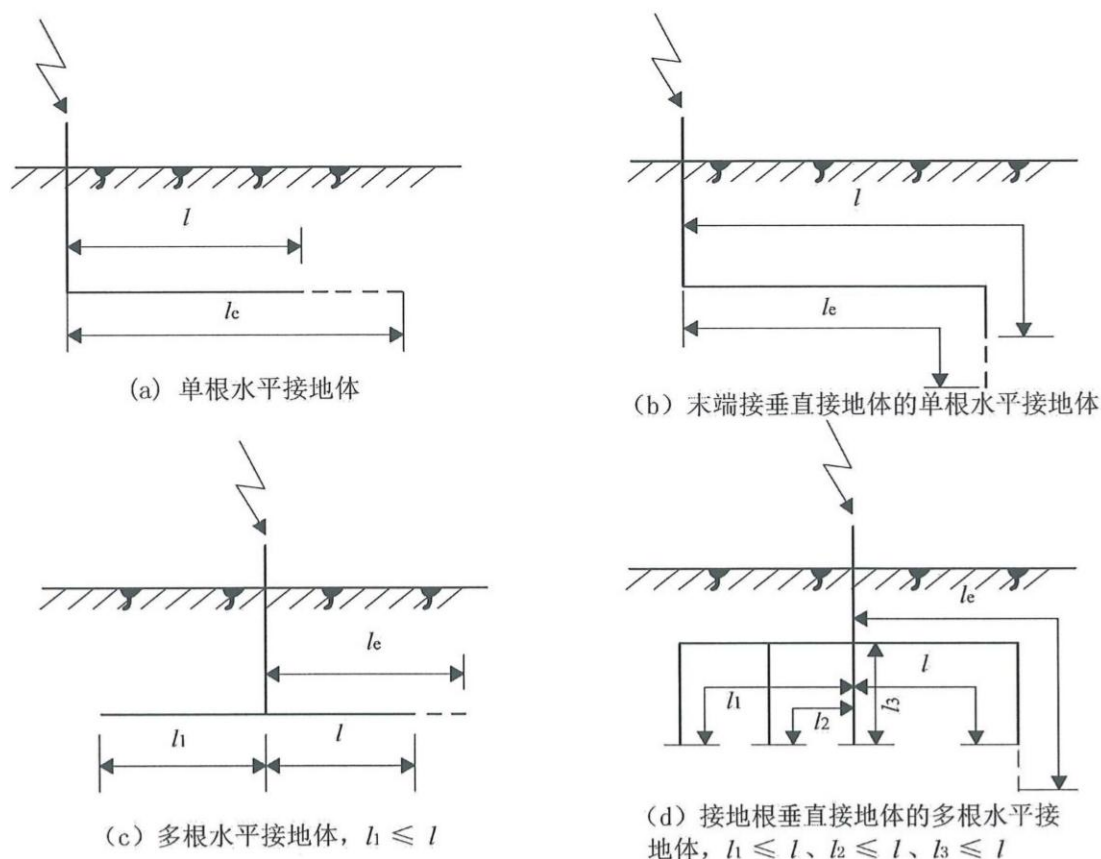
图C.2 接地体有效长度的计量
