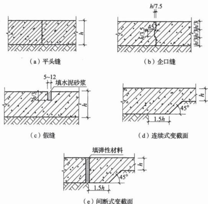
图 6.0.3 混凝土垫层缩缝
