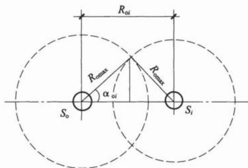
图 C. 2. 10 荷载影响角示意
