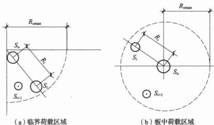
图 C. 2. 9 荷载区域
