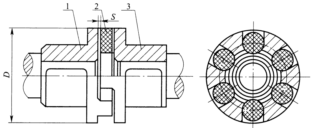
图 5.3.14 梅花形弹性联轴器
