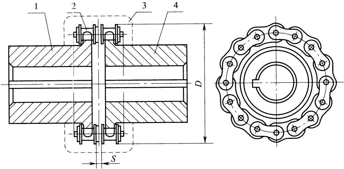
图 5.3.7 滚子链联轴器
