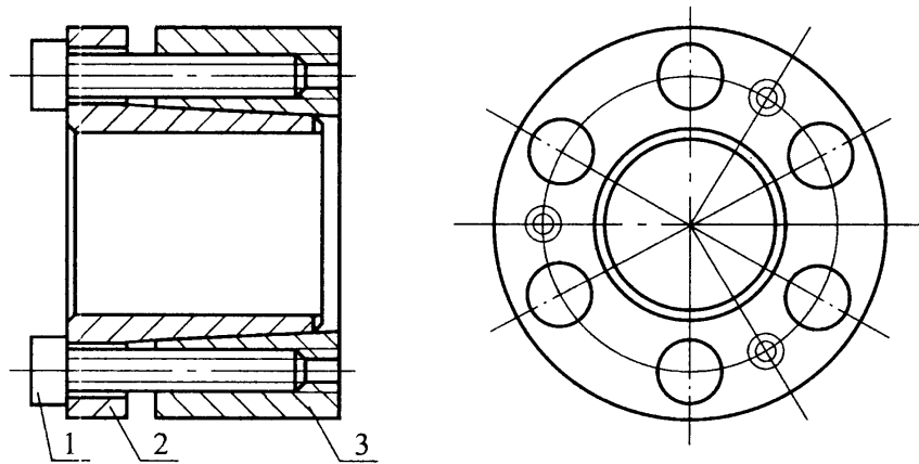
图 5.2.11 胀紧联接套
