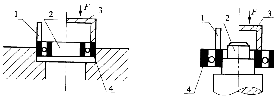
(a) 轴承外圈为固定圈
