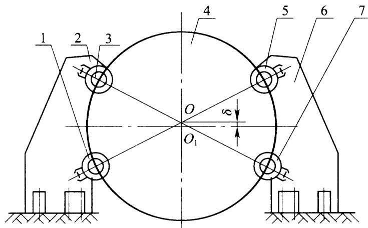
图 5.4.7-2 铅垂面内位置度偏差
