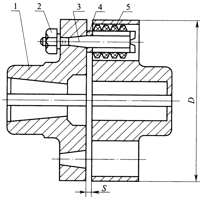
图 5.3.12 弹性套柱销联轴器
