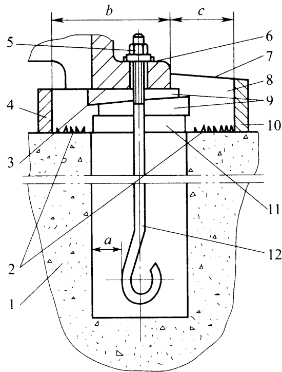
图 4.1.1 安设预留孔中的地脚螺栓
