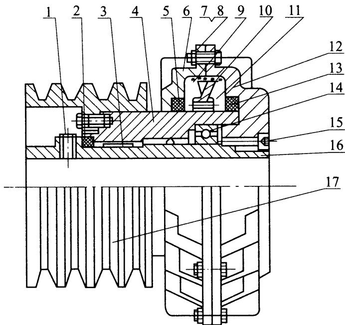
图 5.3.15 V带轮钢砂式安全联轴器
