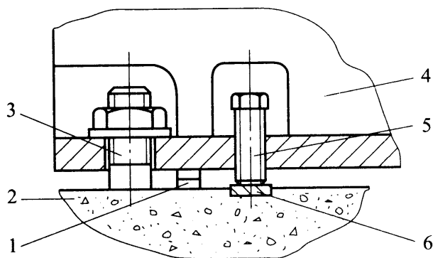
图 4.2.8 调整螺钉
