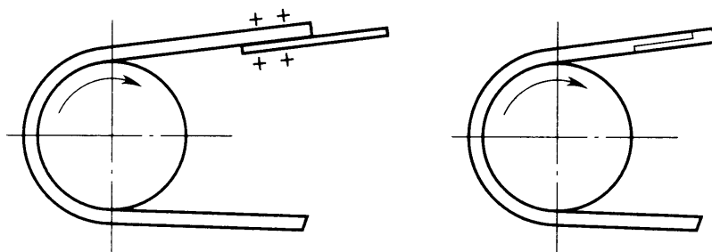
图 5.7.2-2 平带搭接方向与带轮转向
