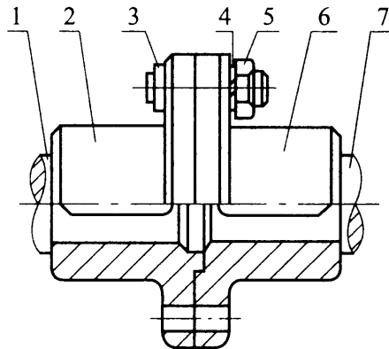
图 5.3.3 凸缘联轴器
