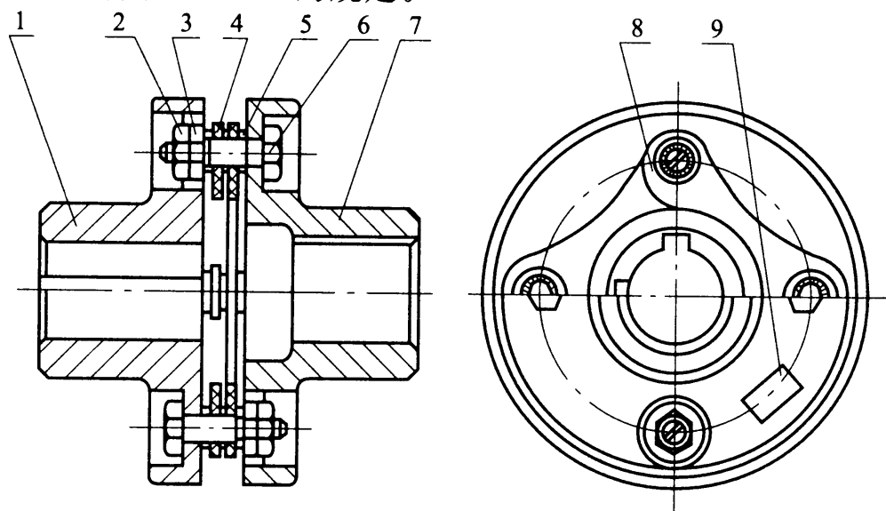
图 5.3.10 膜片联轴器
