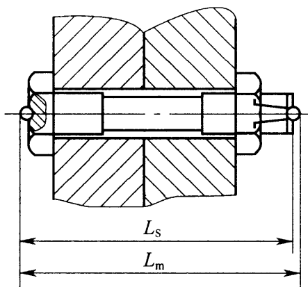
图 5.2.4-1 紧固后的螺栓
