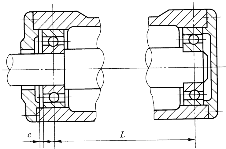
图 5.6.5 向心轴承装配间隙
