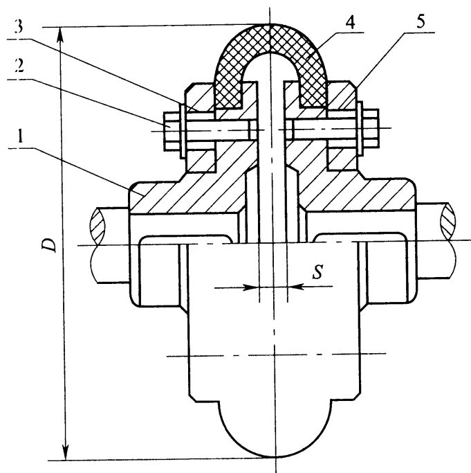
图 5.3.11 轮胎式联轴器
