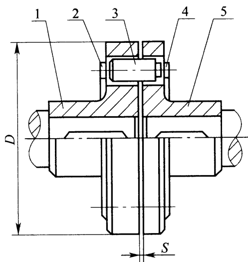
图 5.3.13 弹性柱销联轴器
