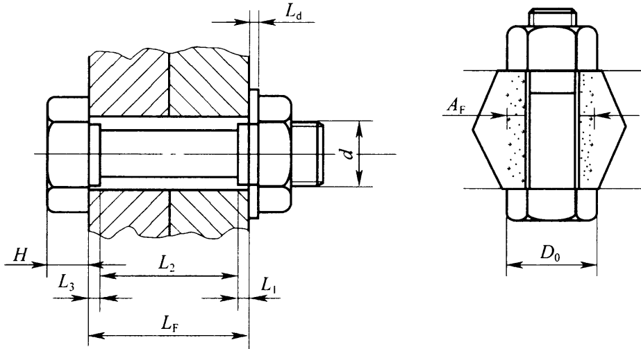
图 F.0.1 螺栓联接
