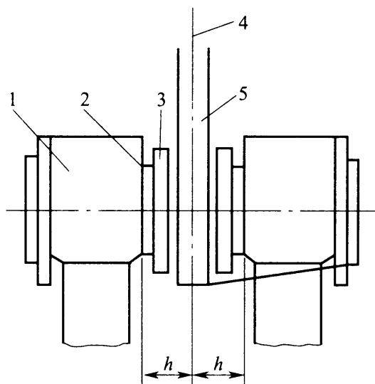
图 5.4.7-1 支架端面与制动盘中心平面间距
