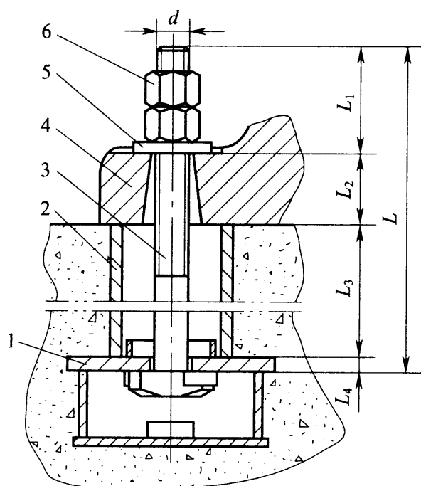
图 4.1.2 安装“T”形头地脚螺栓
