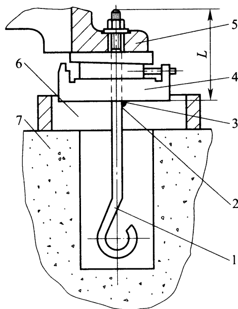
图 C.0.1 压浆法
