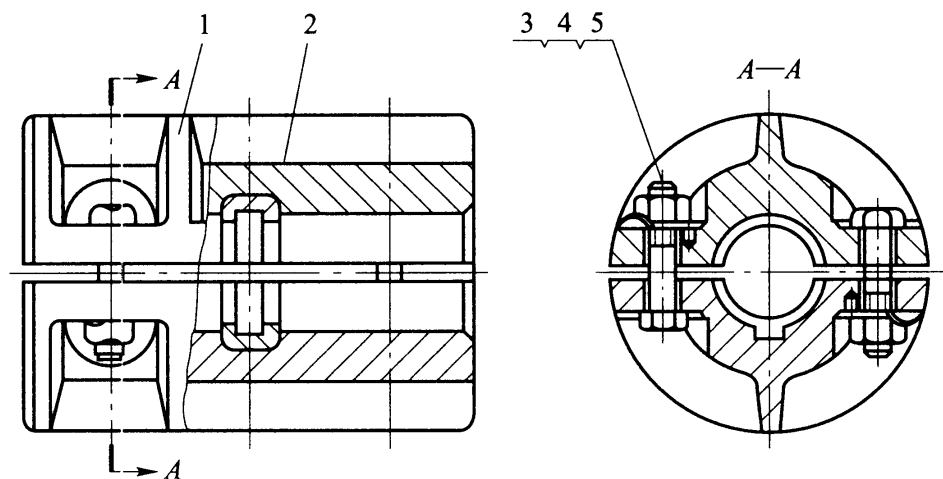
图 5.3.4 夹壳联轴器
