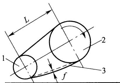
图 5.7.5 传动链条弛垂度
