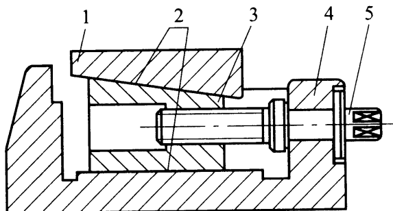
图 4.2.7 螺栓调整垫铁
