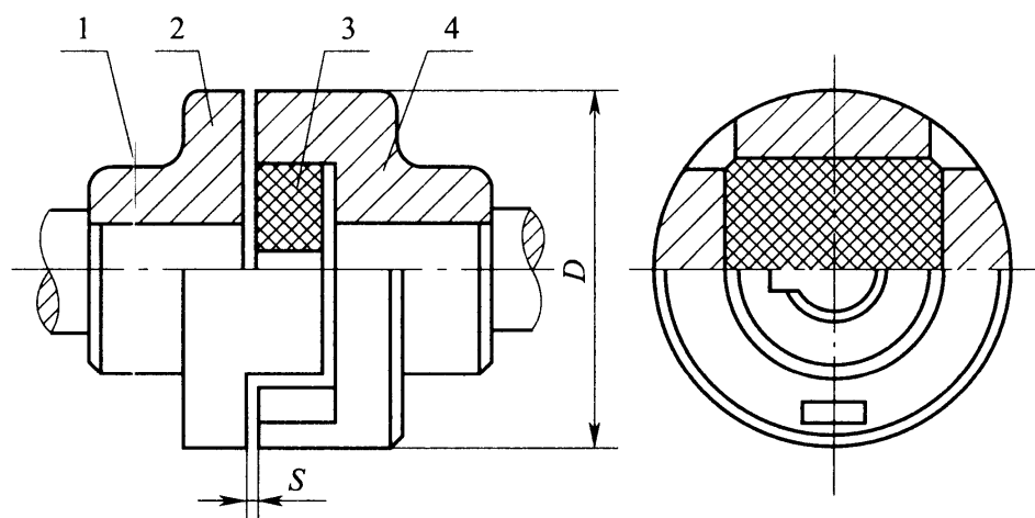
图 5.3.5 滑块联轴器
