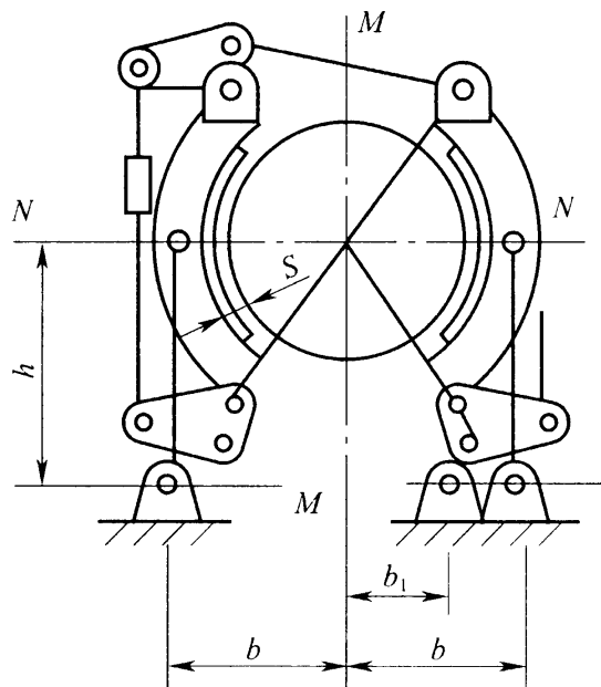
(a) 平移制动器
