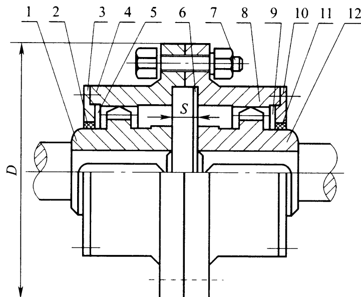
图 5.3.6 齿式联轴器
