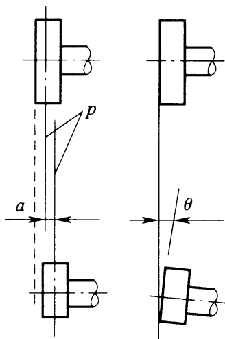
图 5.7.3 两平行带轮的位置偏差
