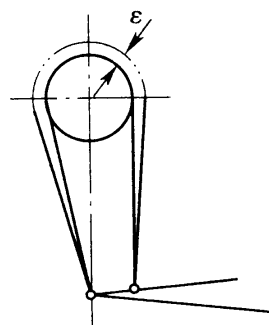
图 5.4.9 带式制动器
