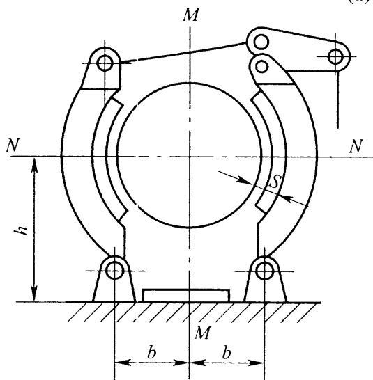
(b) 角移制动器
