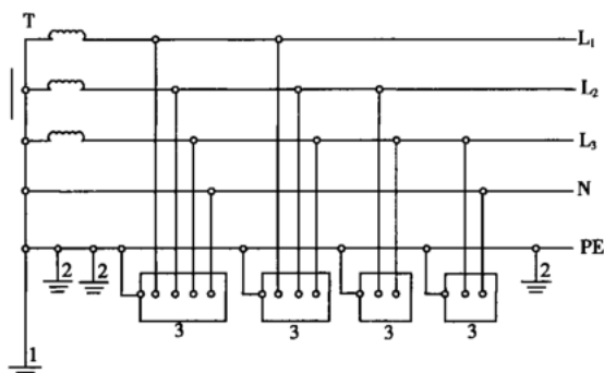
图 4.5.1 专用变压器供电时 TN-S 保护接零系统示意
