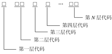
图 1 代码结构
