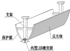
图 3 照明轮廓带组件
