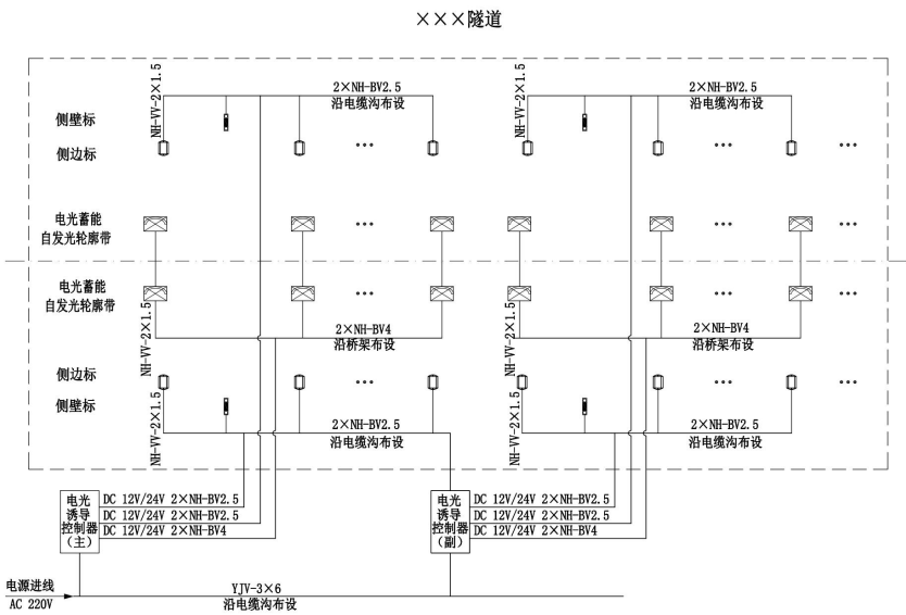
图 C.2 公路隧道弱电供电设施示意图
