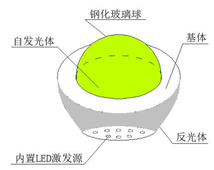
图 7 电光型蓄能自发光突起路标
