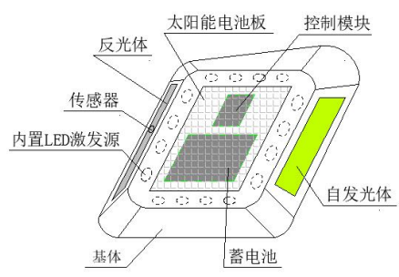
图 8 智能型蓄能自发光突起路标
