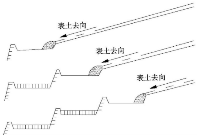
图2 表土逐台下移法
