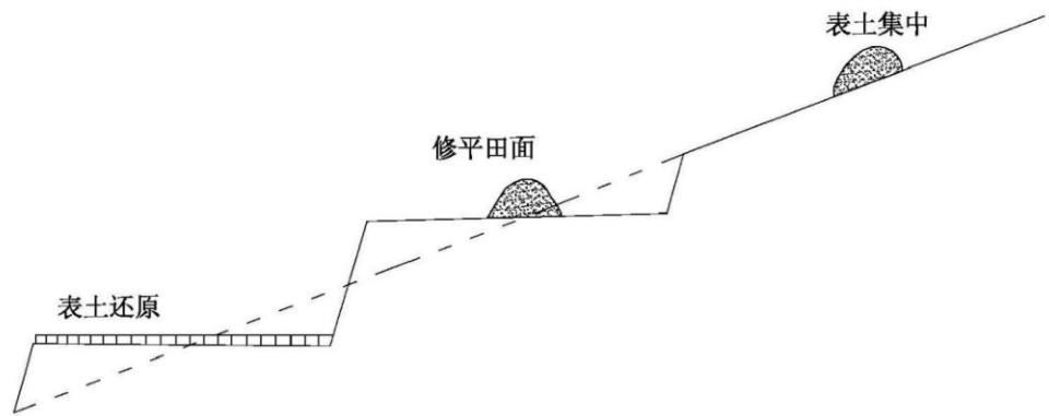
图3 表土中间堆置法
