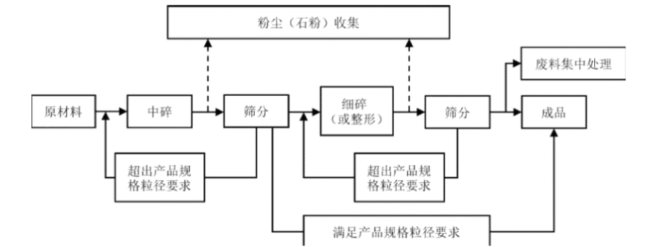
图1 机制砂干法生产工艺流程
