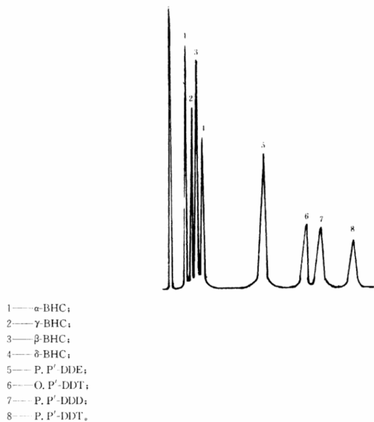
图 1 六六六、滴滴涕气相色谱图
