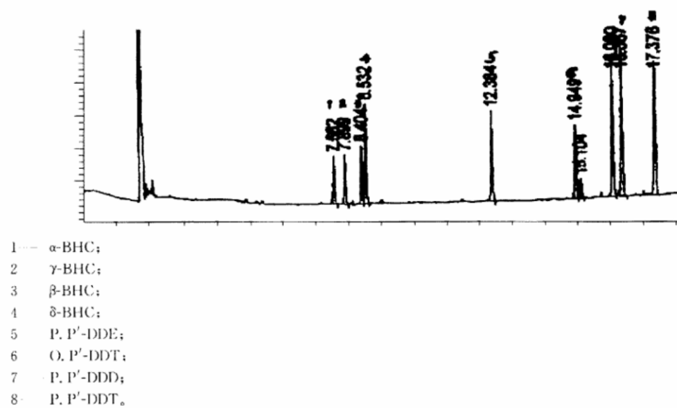
图 2 六六六、滴滴涕气相色谱图
