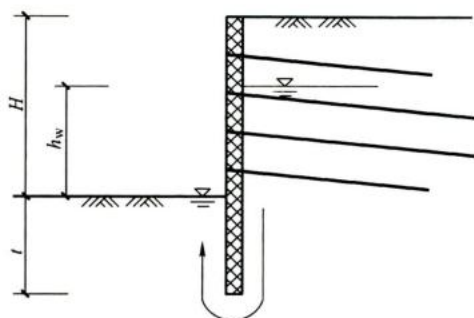
图 4.3.9 抗渗流稳定性验算
