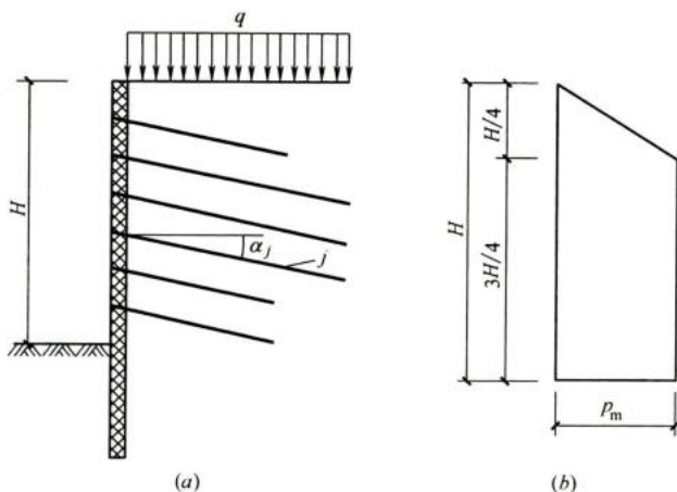
图 4.2.3 土钉轴向荷载标准值计算
