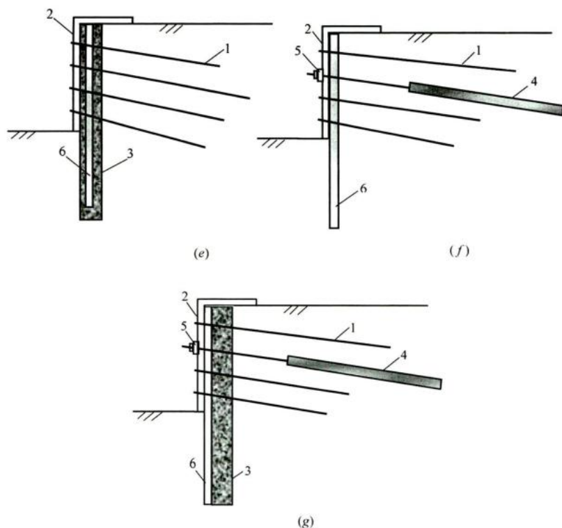
图1 复合土钉墙基坑支护形式(二)
