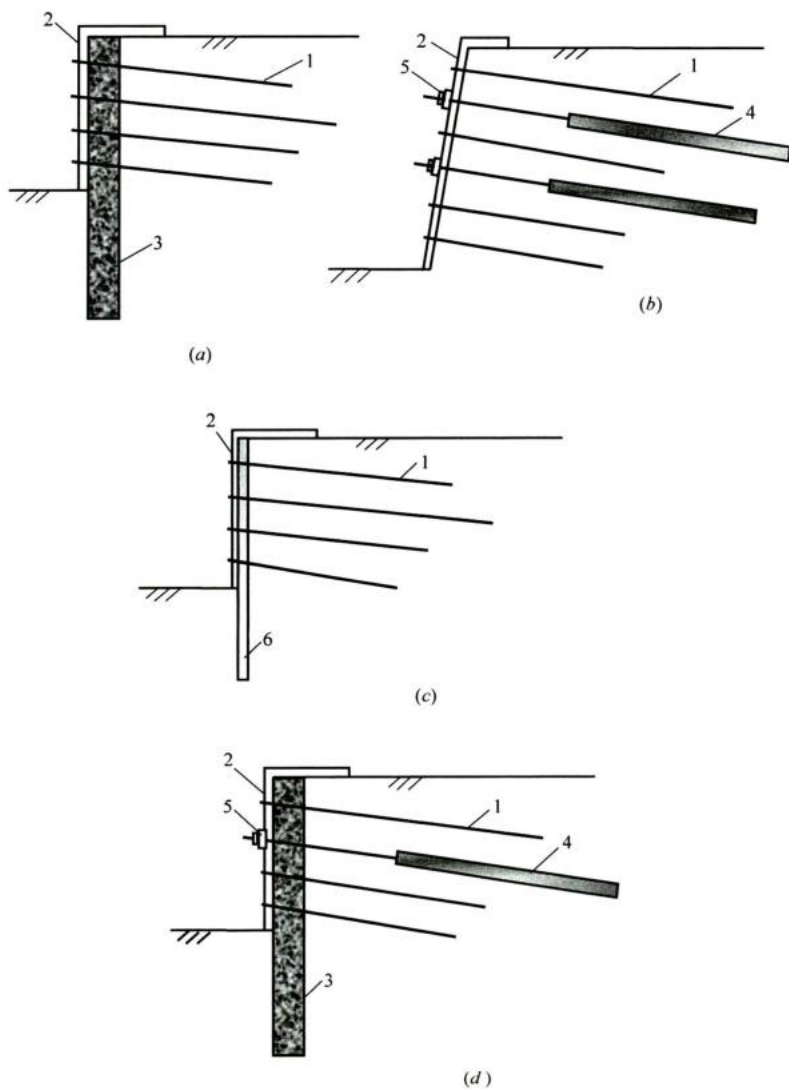
图1 复合土钉墙基坑支护形式(一)
