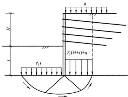
图 4.3.7 坑底抗隆起稳定性验算
