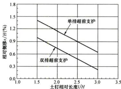
图2 土钉支护位移估算
