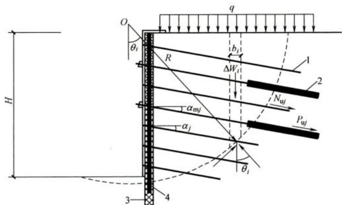
图 4.3.2 复合土钉墙稳定性分析计算
