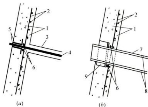
图 4.4.4 土钉与面层连接构造示意
