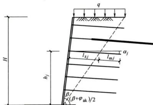
图 4.2.2 土钉长度计算
