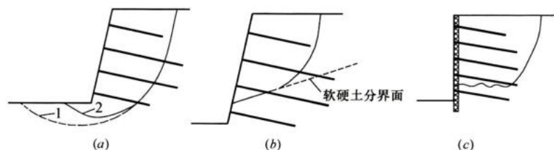
图 4 特殊地质条件下的破坏模式
