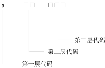
图 1 代码结构图
