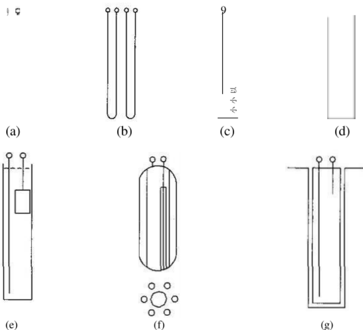
图 3 竖直地埋管换热器形式
