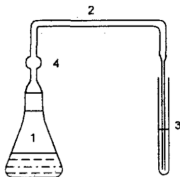
砷化氢发生与吸收装置图
