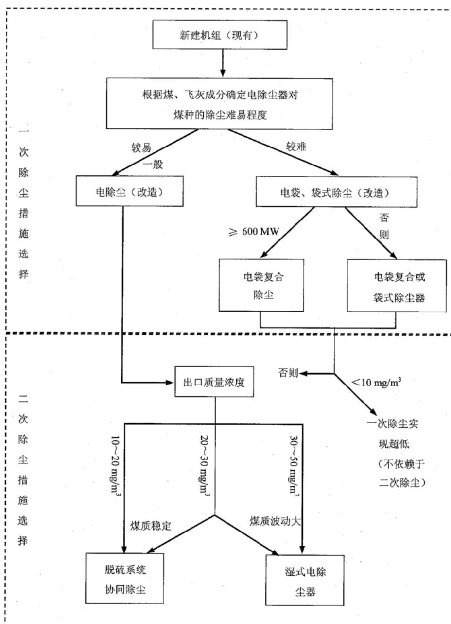
图 1 颗粒物超低排放技术路线
