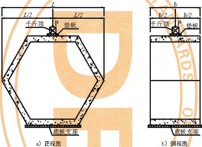
图E.1 加载示意图
