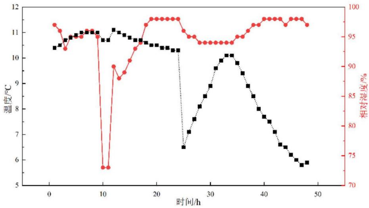
图F.11 C 项目温度和湿度记录图
