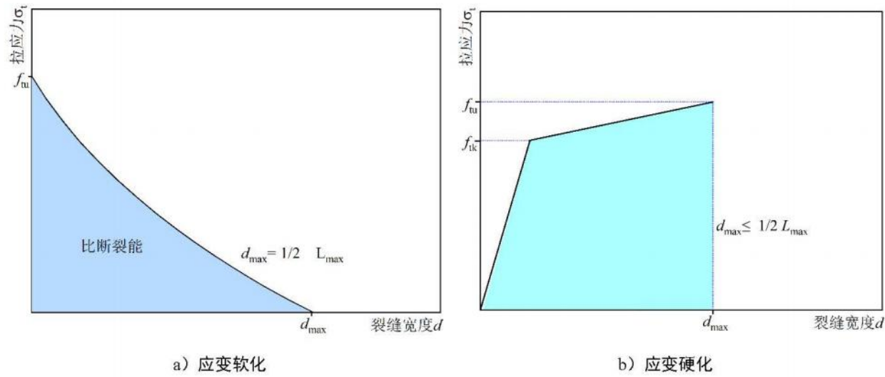
图F.1 拉应力与最大裂缝宽度示意图
