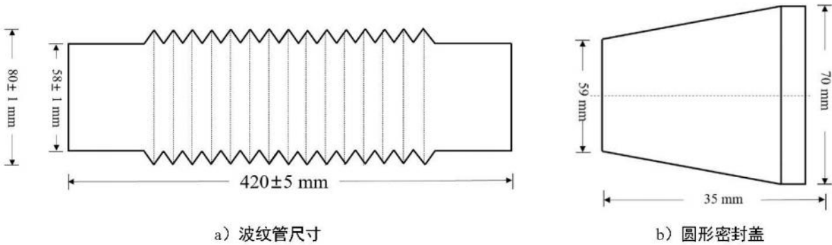
图C.1 超高性能混凝土早龄期收缩模具尺寸
