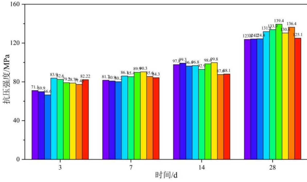
图F.7 B 高速项目抗压强度数据
