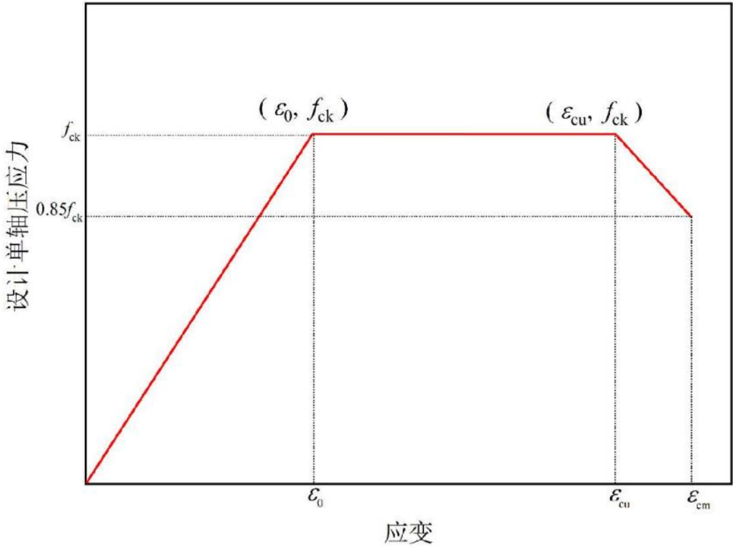
图A.1 单轴受压应力-应变关系
