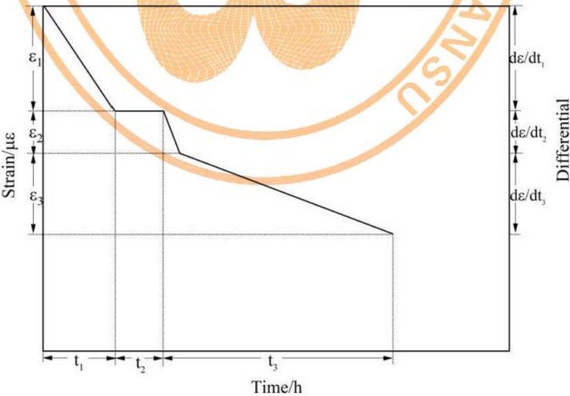
图C.2 超高性能混凝土早龄期自收缩示意图
