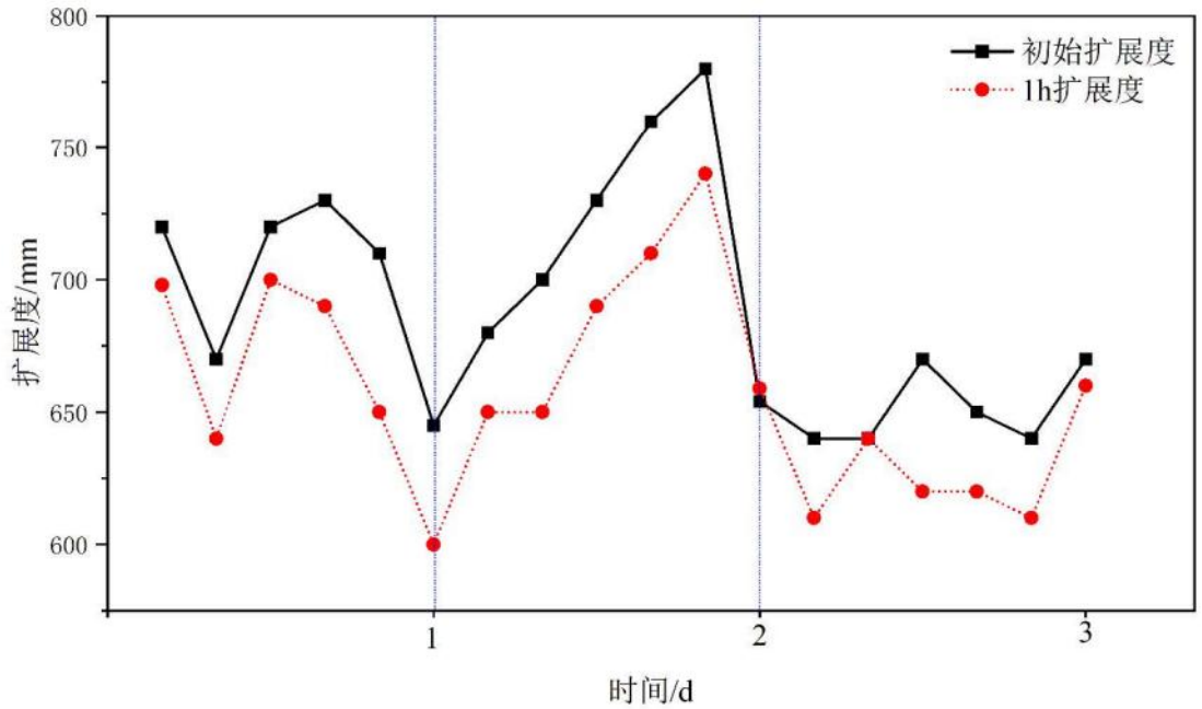
图F.3 A 高速扩展度数据
