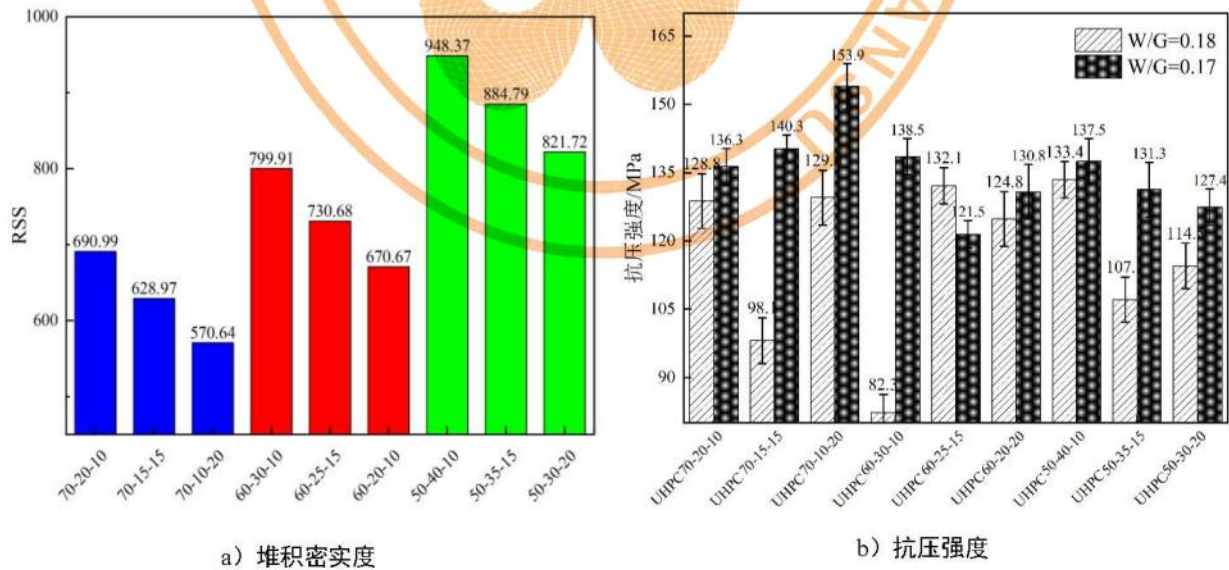
图F.17 最紧密堆积模型抗压强度验证
