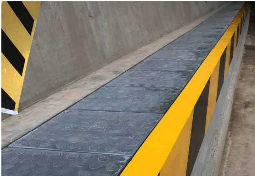
图F.18 超高性能混凝土隧道电缆槽盖板应用
