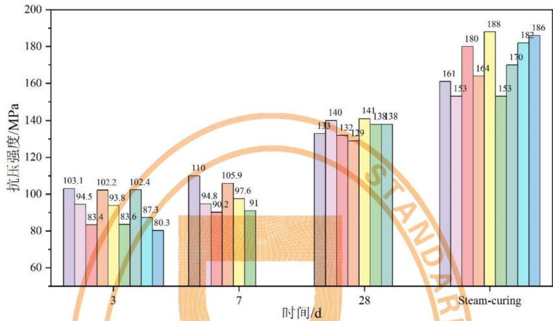
图F.4 A 高速抗压强度数据
