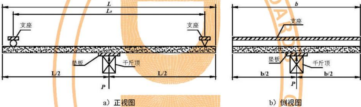
图D.1 加载示意图 1
