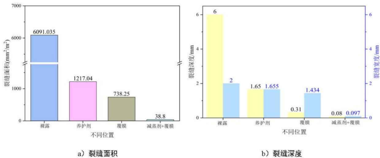
图F.10 不同养护位置裂缝情况
