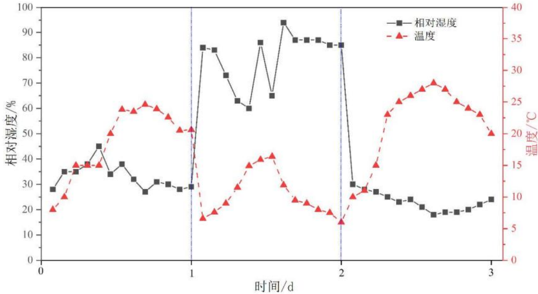
图F.2 A 高速温度和湿度记录图
