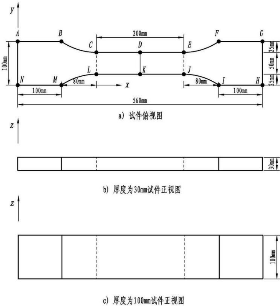
图B.1 抗拉性能测试试件尺寸示意图
