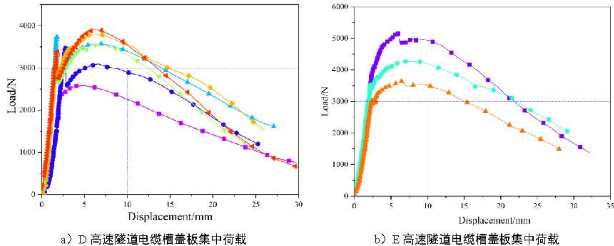
图F.19 超高性能混凝土隧道电缆槽盖板集中荷载
