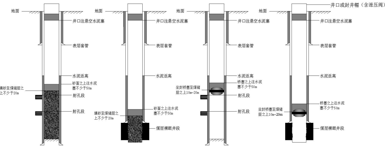
1) 套管完井水泥塞封层 2) 裸眼完井水泥塞封层 3) 套管完井桥塞封层 4) 裸眼完井桥塞封层
