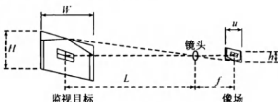
图 1 光学成像关系图
