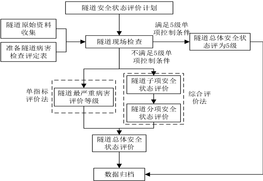
图 1 盾构隧道安全评价流程
