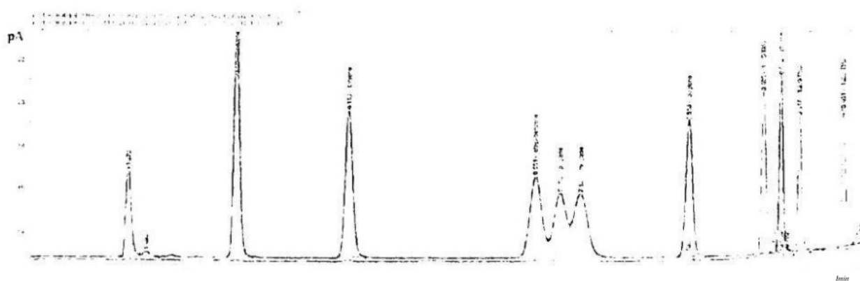
图D.1 苯、甲苯、乙苯、对-二甲苯、间-二甲苯、邻-二甲苯、1,3,5-三甲苯、苯乙烯、1,2,4-三甲苯和1,2,3-三甲苯色谱图
