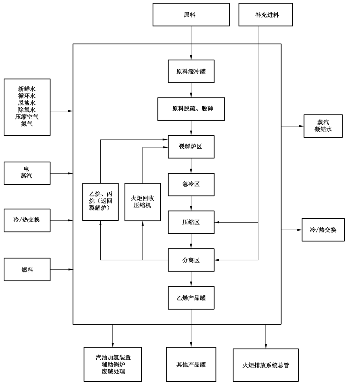
图 B.1 乙烯装置能耗统计界区图
