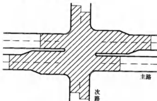
图 2 交叉口范围示意图
