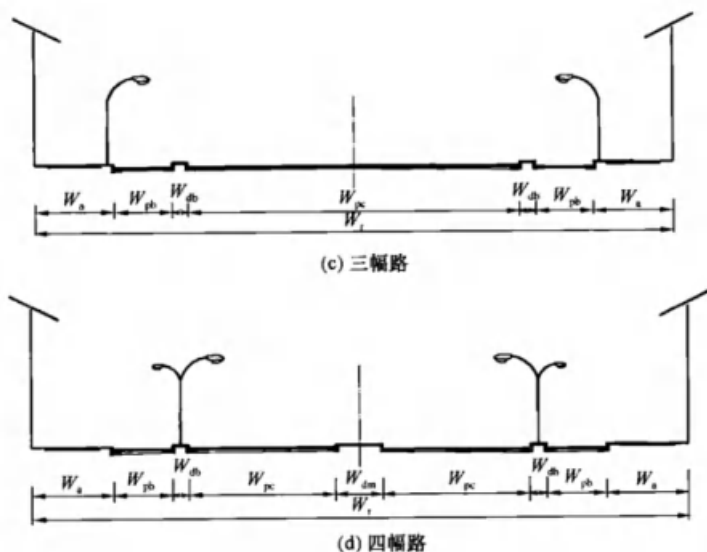
图 5.2.1 横断面形式
