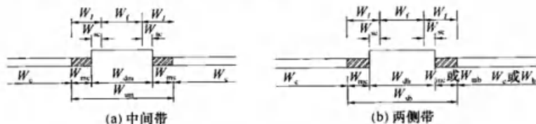
图 5.3.5 分车带
