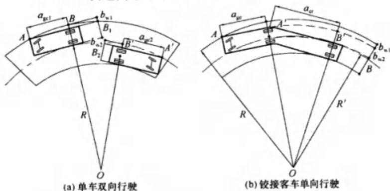
图 1 圆曲线上路面加宽示意图
