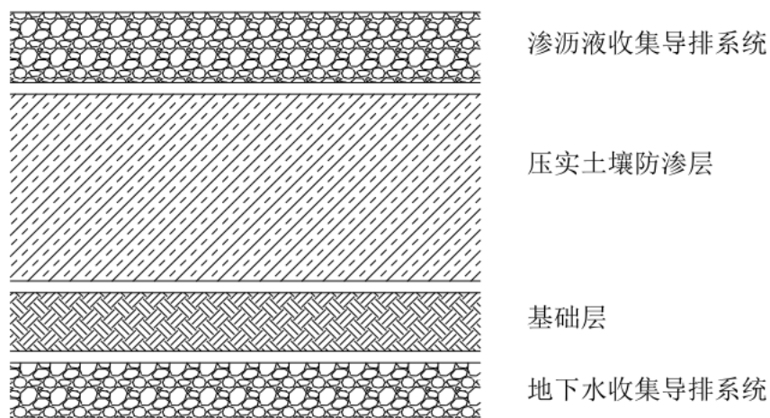
图 3.2.2-3 压实土壤单层防渗结构示意图
