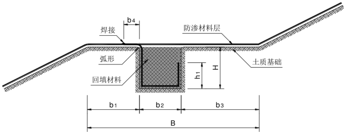
图 3.7.4-1：边坡锚固平台典型结构图
