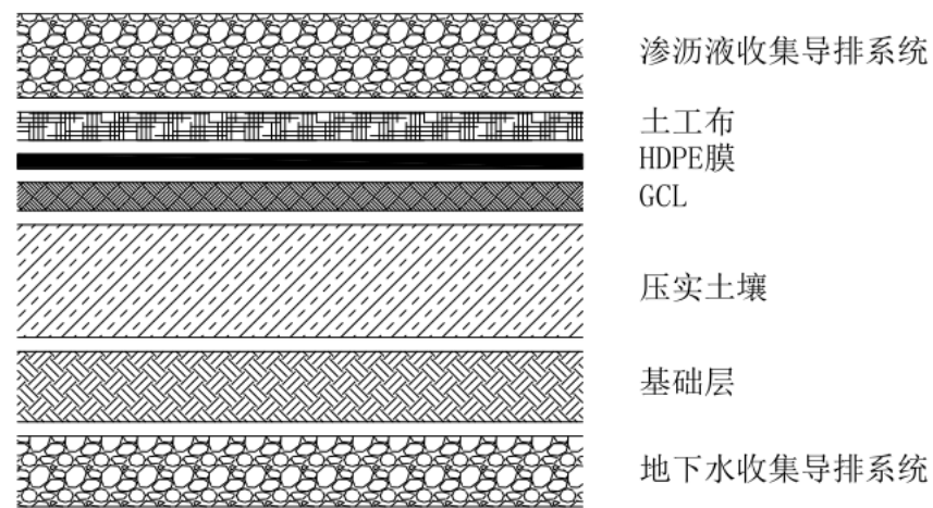
图 3.2.2-2 HDPE 膜+GCL 复合防渗结构示意图
