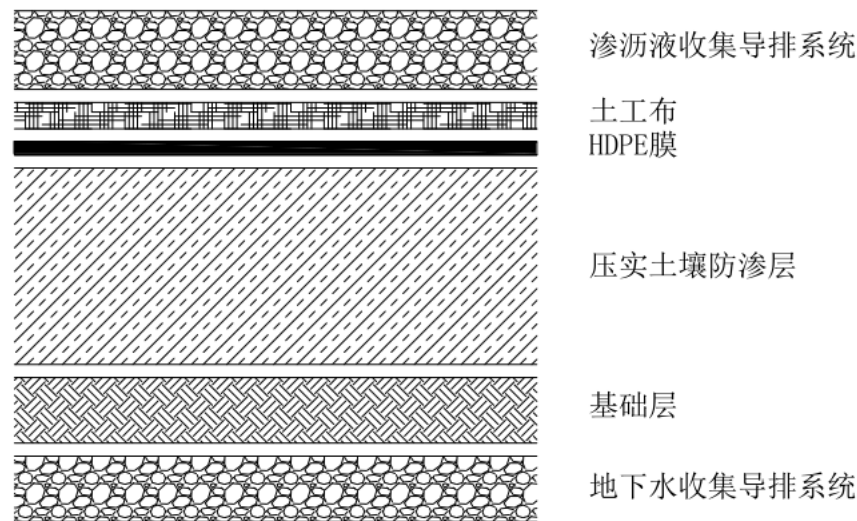
图 3.2.2-1 HDPE 膜+压实土壤复合防渗结构示意图
