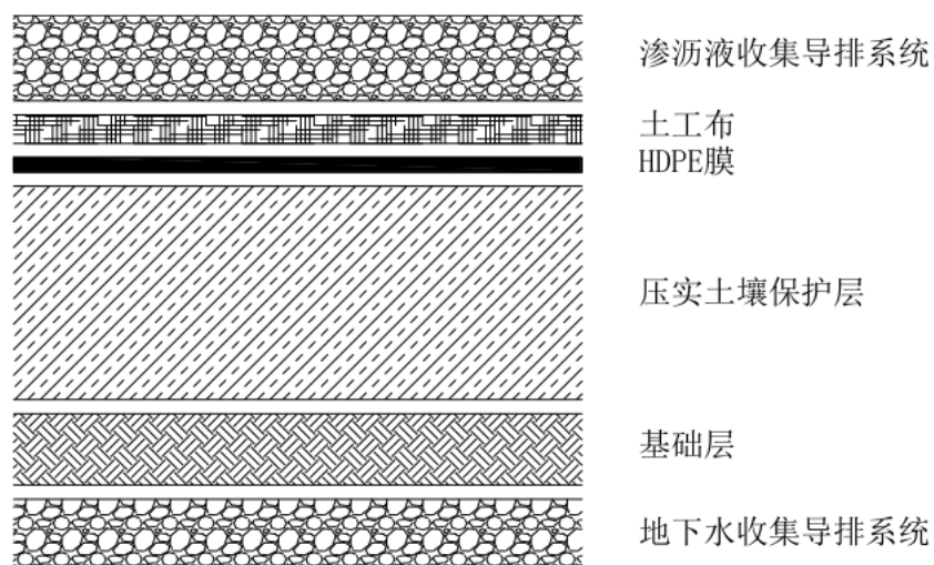
图 3.2.2-4 HDPE 膜单层防渗结构示意图
