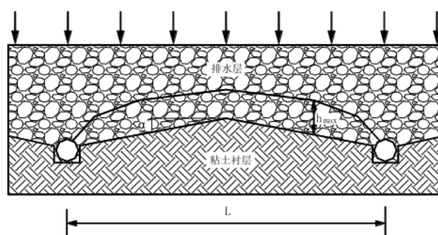
图 3.1.5 最大渗沥液水头示意图
