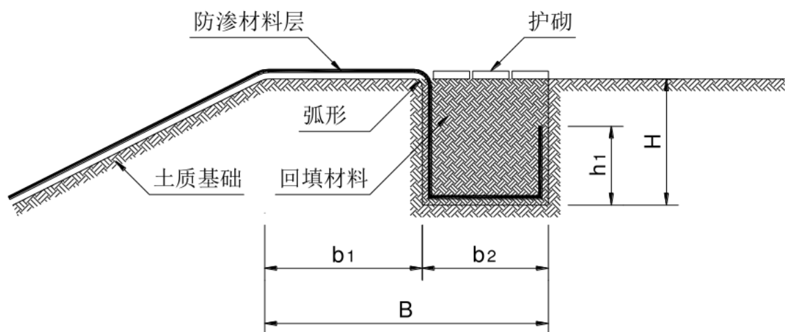
图 3.7.4-2：终场锚固沟典型结构图
