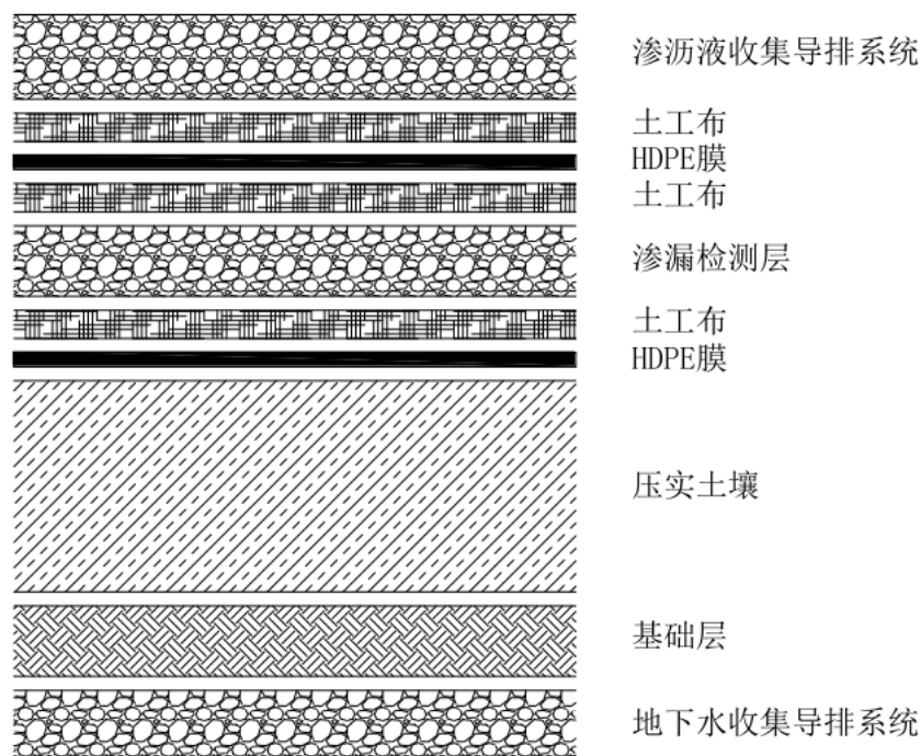
图 3.2.2-2 双层防渗结构示意图
