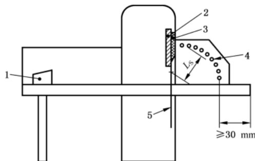
图 2 切纸机前部联锁防护装置(侧面视图)
