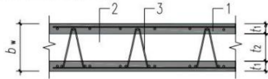
图 10.3.1-6a 双面叠合剪力墙构造
