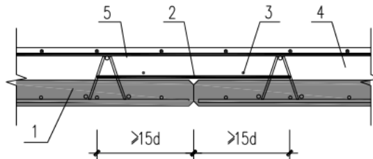
图 10.6.6 单向板板侧分离式拼缝构造示意
