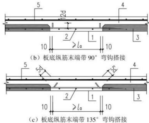
图 10.6.7 双向叠合板整体式拼缝构造示意
