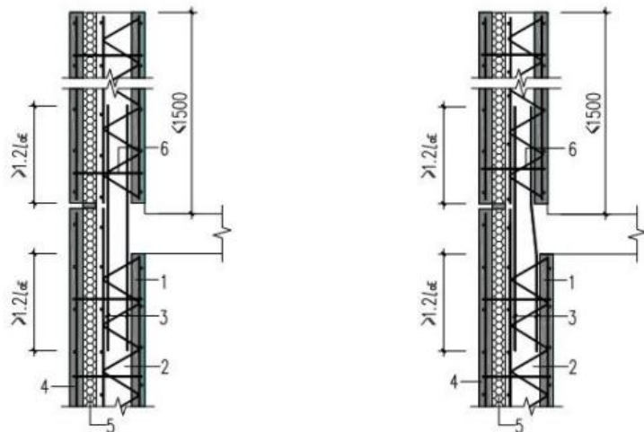
(c) 叠合剪力墙与叠合女儿墙（等厚） (d) 叠合剪力墙与叠合女儿墙（不等厚）
