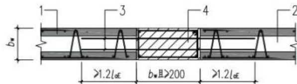
(a) 连接构造（一）
