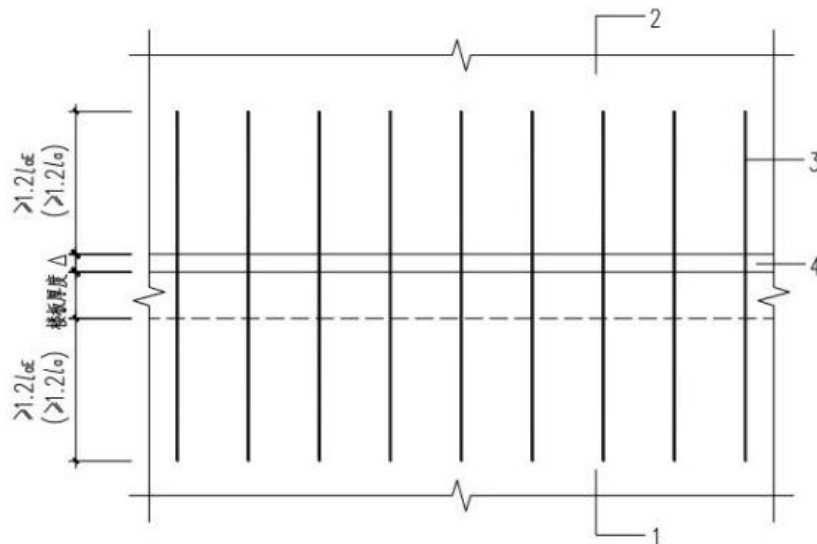
图 10.4.4 竖向连接钢筋搭接构造
