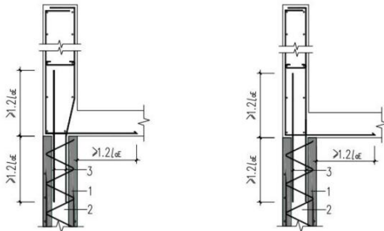
(a) 叠合剪力墙与现浇女儿墙（等厚）
