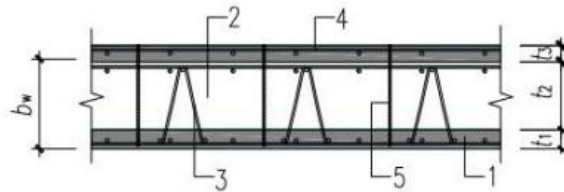
图 10.3.1-6a 双面叠合剪力墙构造
