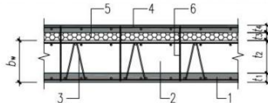
图 10.3.1-6b 单面叠合剪力墙构造（无夹芯保温层）
