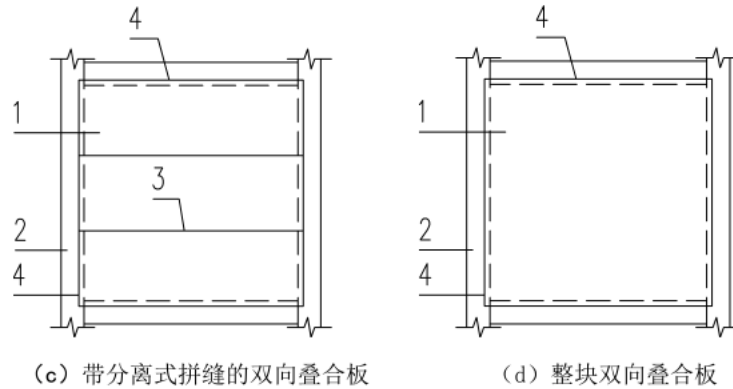
图 10.6.5 预制叠合板形式
