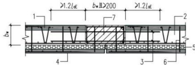
图 10.5.3 单面叠合剪力墙竖向接缝连接构造
