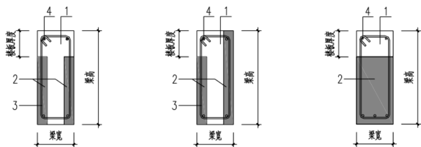
(a) 叠合连梁 (构造 1)
