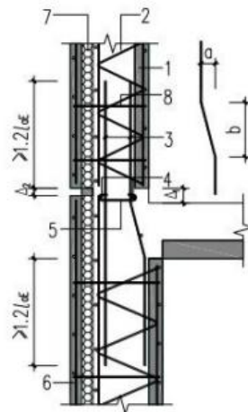
(d) 叠合剪力墙 (不等厚, a/b \leq 1/6 )
