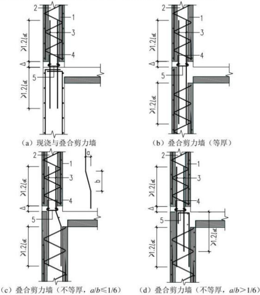
图 10.4.7 双面叠合剪力墙水平接缝连接构造
