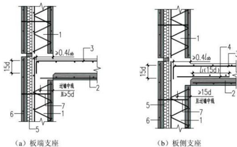
图 10.6.9-1 双面叠合剪力墙与叠合楼板连接节点构造示意
