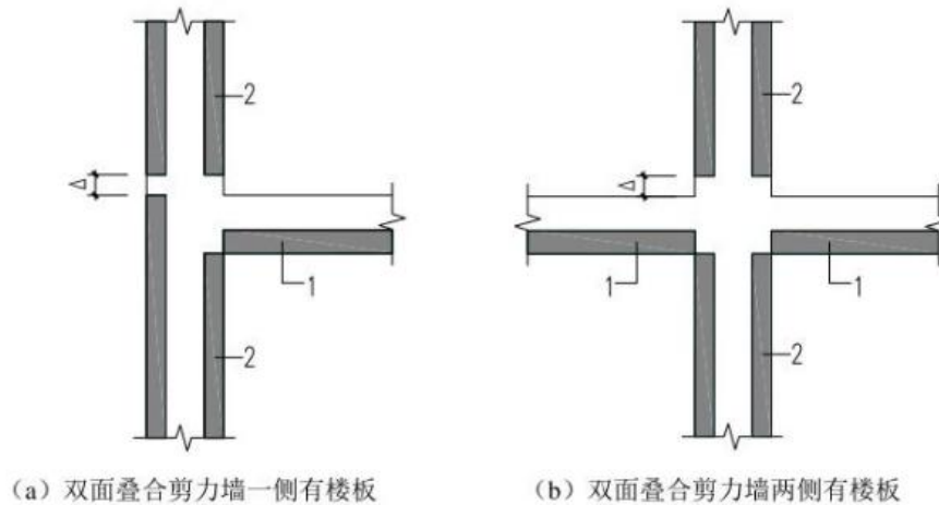
图 10.4.3 双面叠合剪力墙水平接缝高度要求 ( 50\text{mm} \leq \Delta \leq 100\text{mm} )
