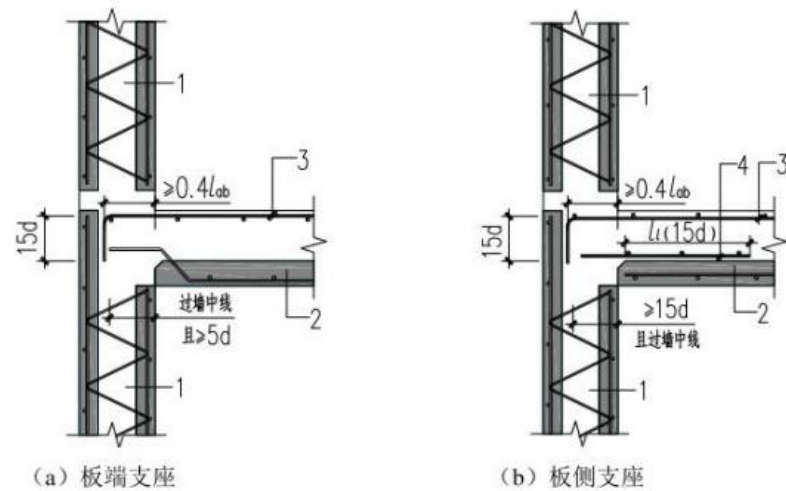
图 10.6.9-1 双面叠合剪力墙与叠合楼板连接节点构造示意
