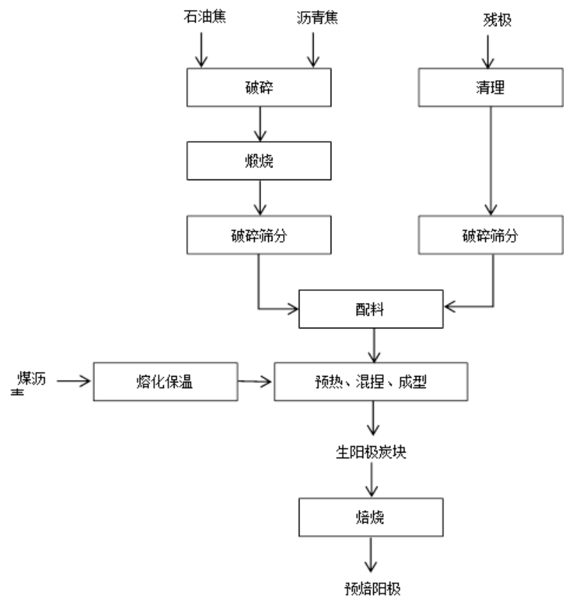
图A.2 预焙阳极生产工艺流程图
