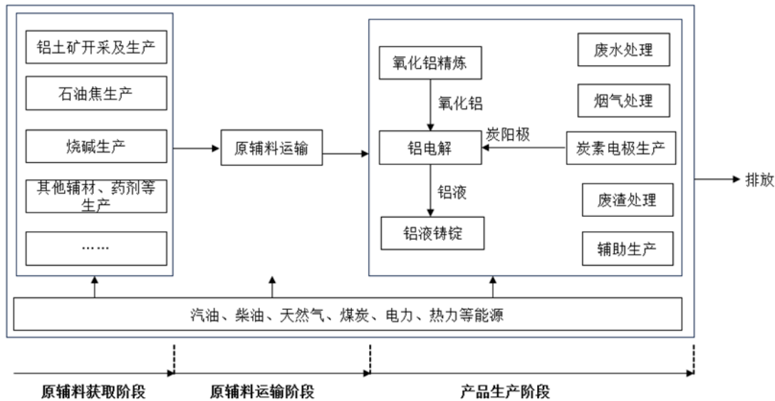
图1 电解铝产品碳足迹评价系统边界示意图
