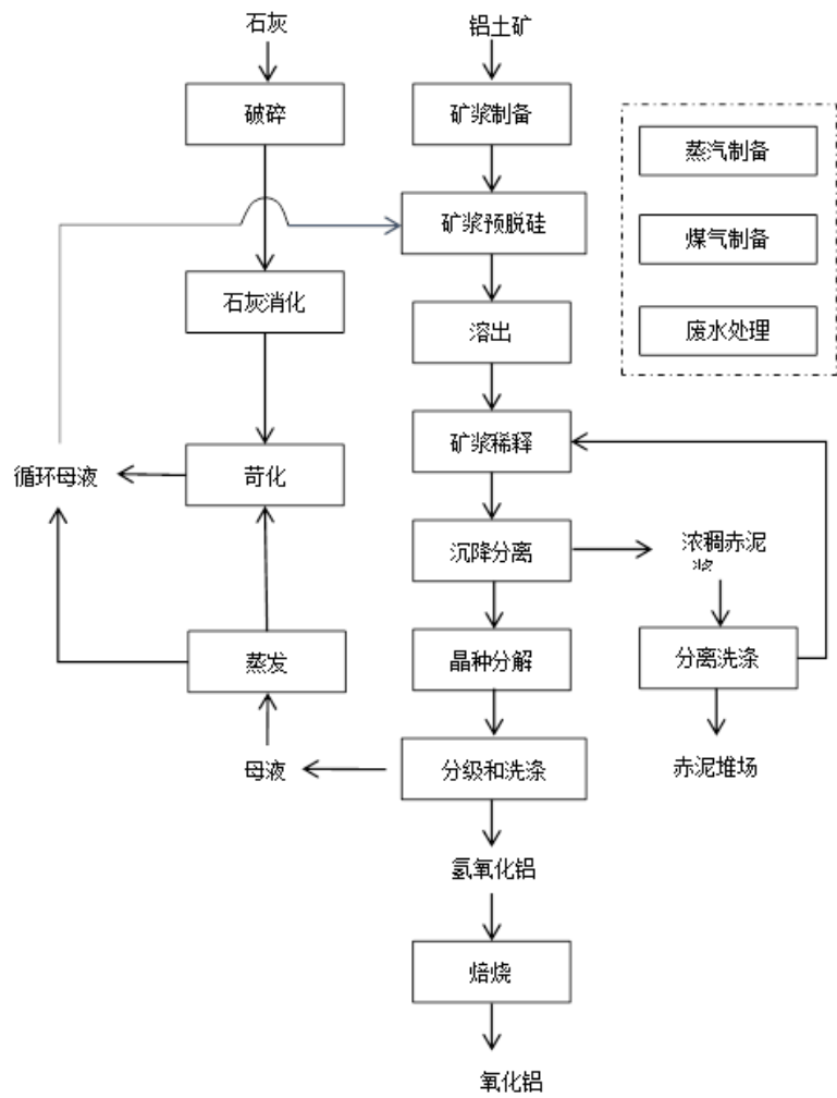
图A.1 拜耳法生产氧化铝工艺流程图
