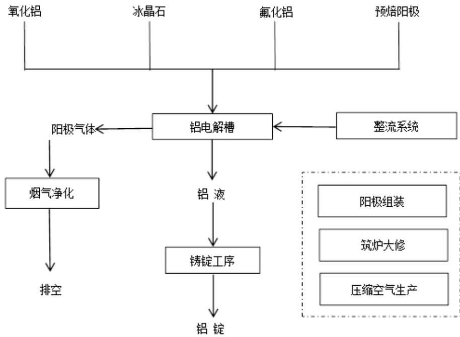
图A.3 铝电解生产与铸锭工艺流程图
