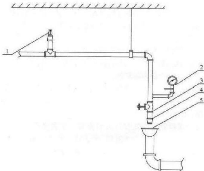
图3 末端试水装置图
