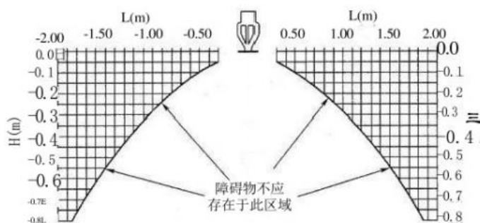
图5.2.12 喷头与障碍物的相对位置
