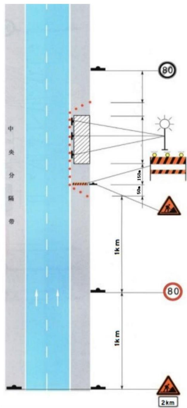
图B. 1 施工作业控制区布置
