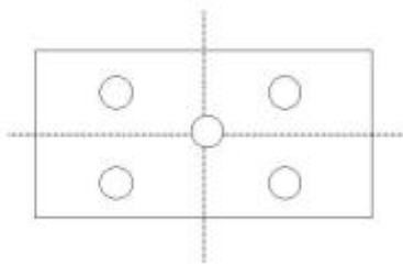
图 C.1 小截面风口测点布置
