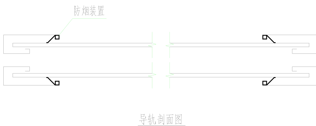
图 D.1 防火卷帘门嵌入深度和内幅宽图示
