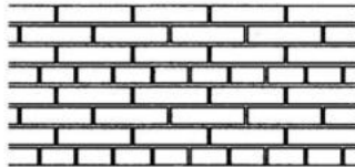
(d) 三顺一丁砌法
