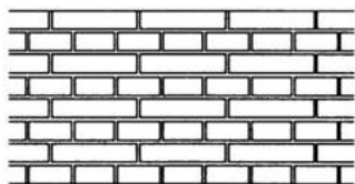
(a) 一顺一丁的十字缝砌法
