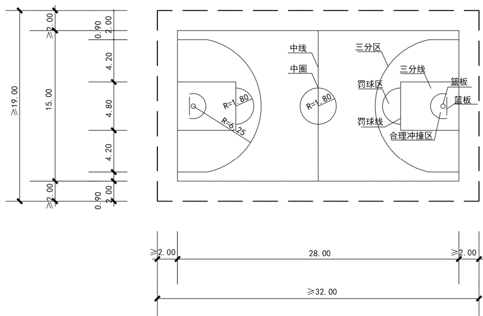
图9 中小学校篮球场尺寸示意图
