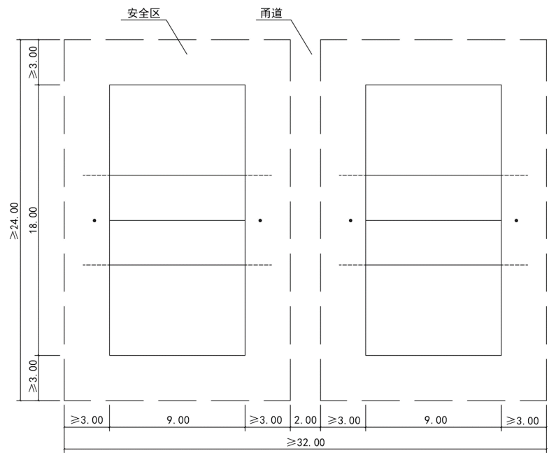
图 13 中小学校排球场地横向排列平面图
