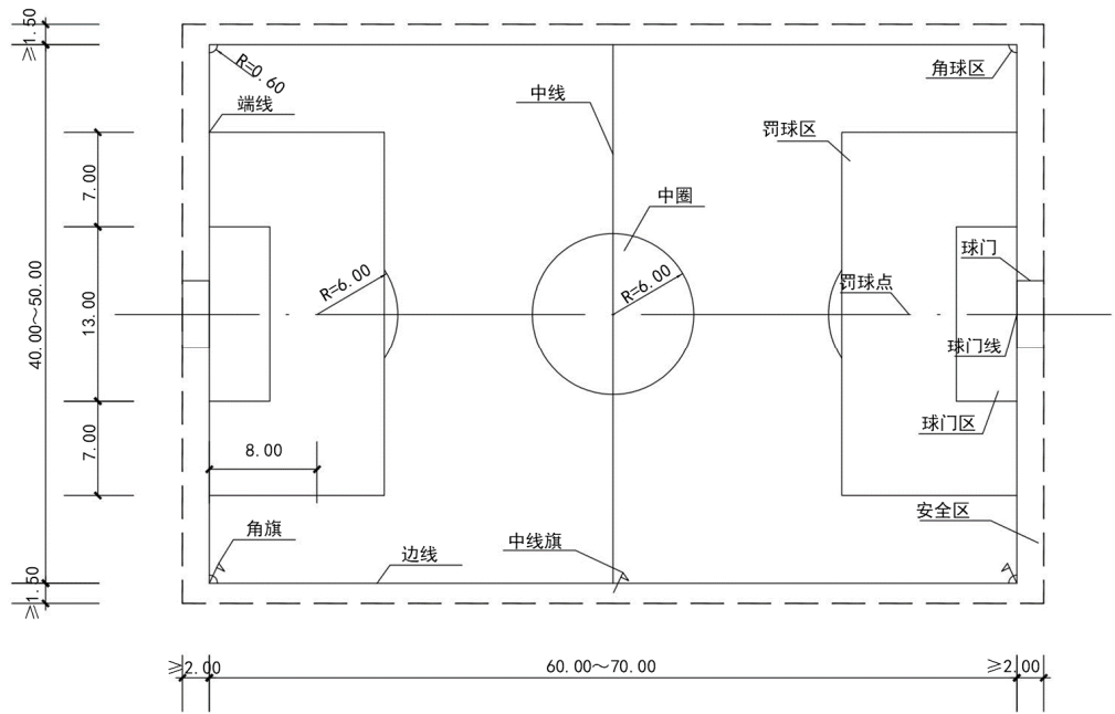
图 7 8 人制（7 人制）足球场地示意图
