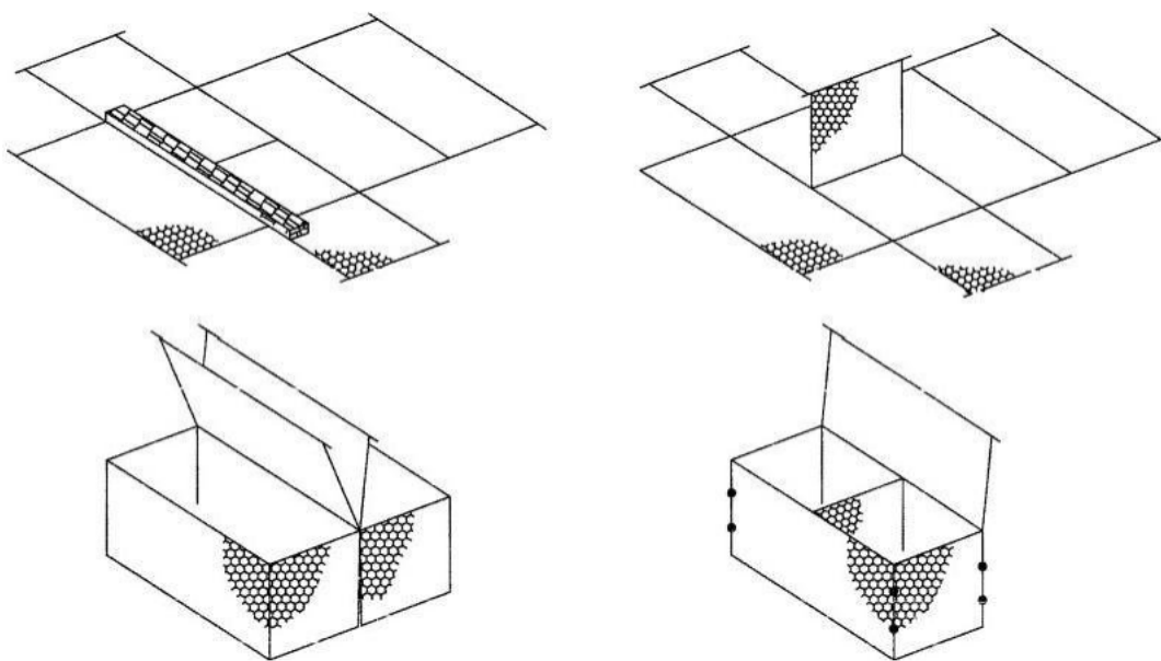
图 3 固滨笼组装示意
