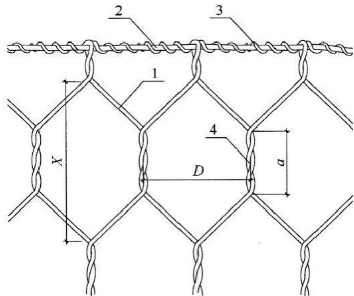
1—网丝；2—边丝；3—机械收边；4—网丝机械绞合： a—绞合长度
