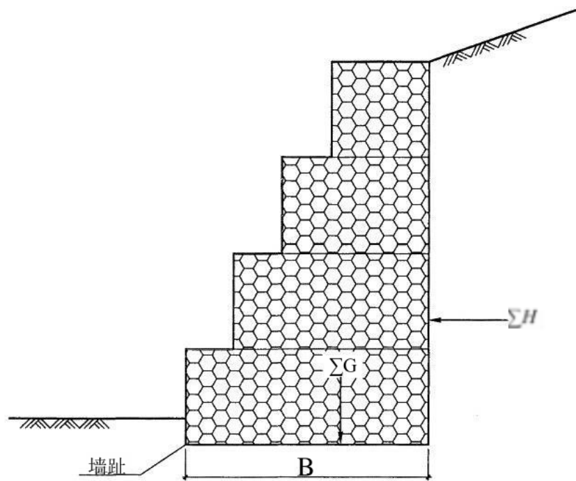
图5.2.3 固滨笼挡土墙稳定性计算简图
