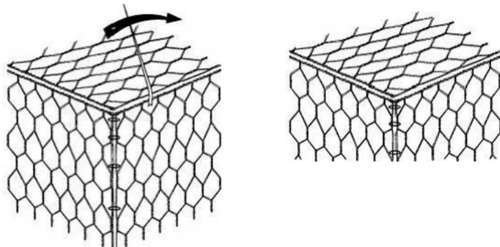
图7.2.1-2 箱体封盖示意
