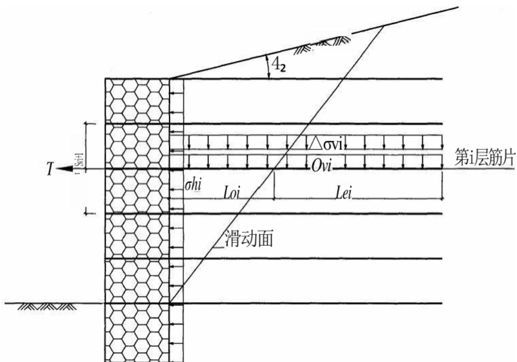
图5.3.2 加筋固滨笼挡土墙剖面示意图
