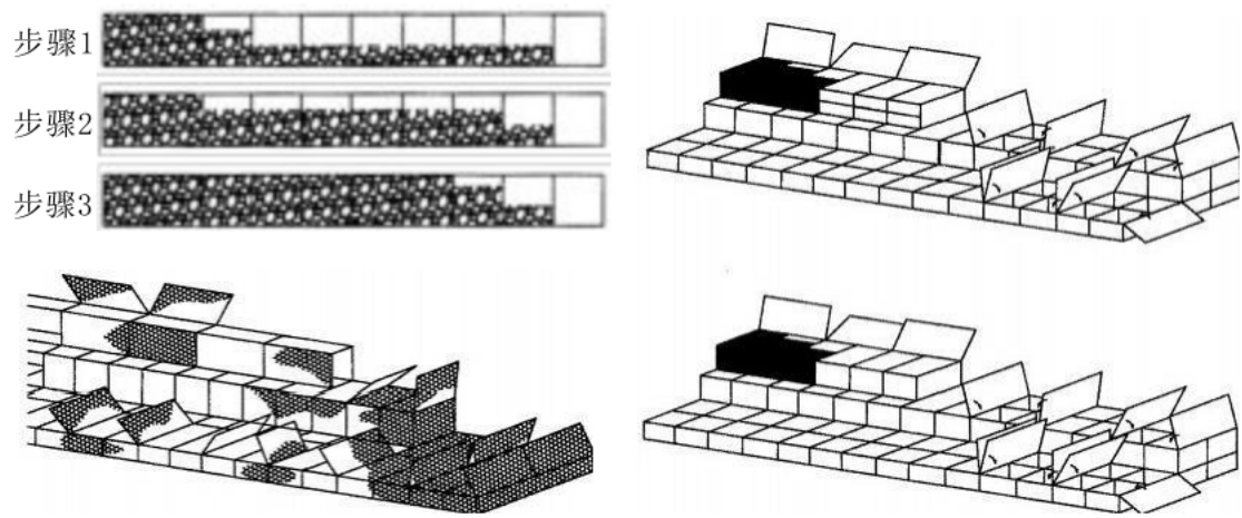
图 4 固滨笼组合体填料示意
