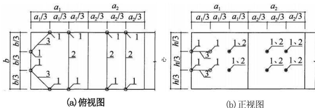
图7.3.4 固滨笼内部连接加强钢丝及绑扎示意
