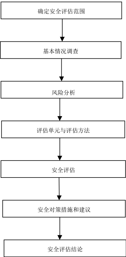
图1 安全评估工作程序框图
