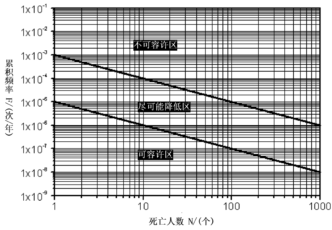
图D.1 可容许社会风险标准 ( F-N ) 曲线
