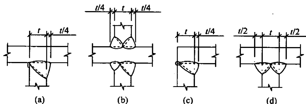
图 6.4.1 焊脚尺寸
