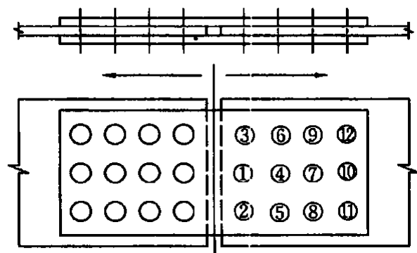
图 1 一般节点施拧顺序
