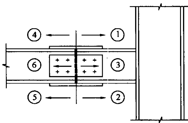
图 3 工字梁节点施拧顺序
