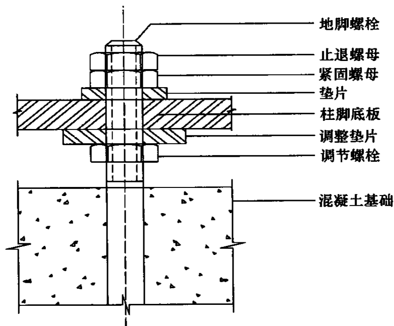
图4 柱脚底板标高精确调整
