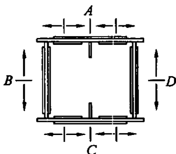
图 2 箱形节点施拧顺序
