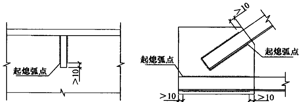
图 6.4.6 起熄弧点位置
