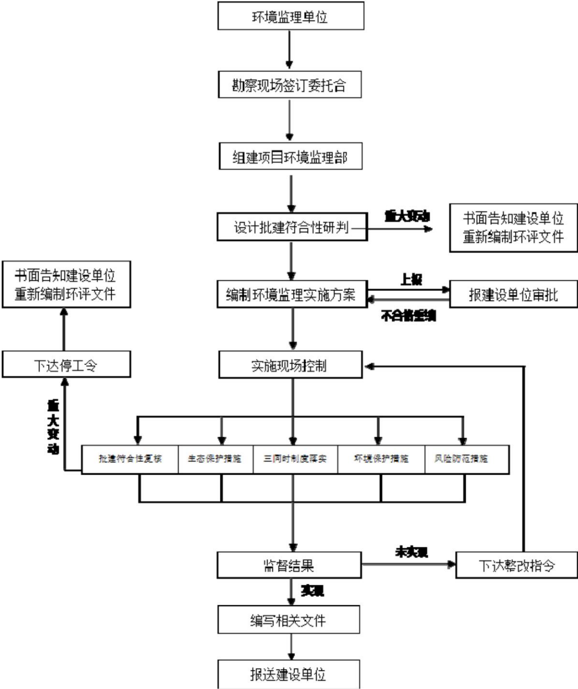
图A. 1 环境监理工作流程图
