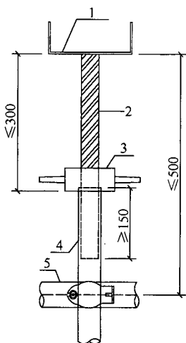
图 1 扣件式钢管支架
