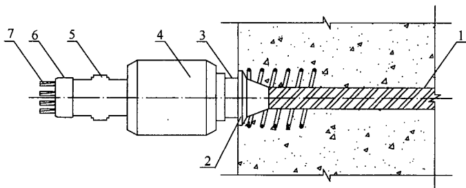
图 E.0.1 摩擦损失测试设备安装示意
