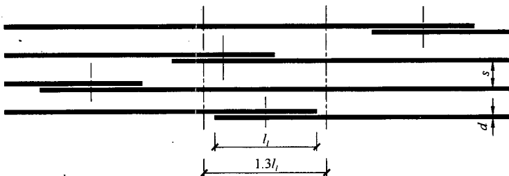
图 5.4.5 钢筋绑扎搭接接头连接区段及接头面积百分率
