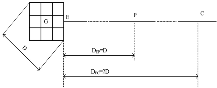
图 A.3 补偿法
