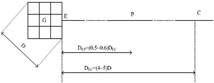
图 A.2 直线法
