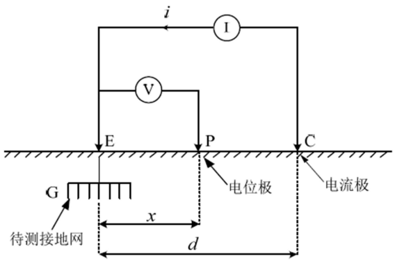
图 A.1 电位降法接线原理图
