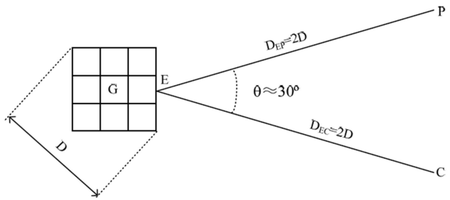
图 A.4 三角法
