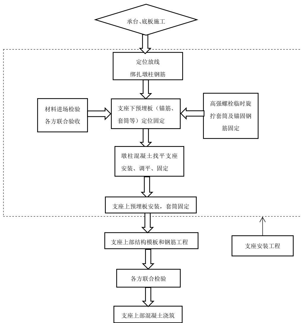
图 5 支座安装的施工流程
