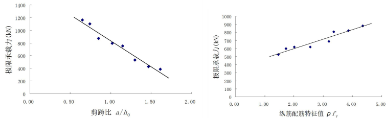
(a) a/h_0 对节点承载力的影响 (b) 托换梁纵筋配筋特征值对节点承载力的影响
