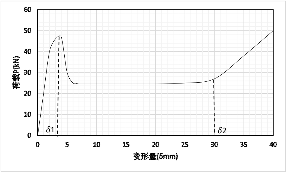
图A. 1 典型荷载-位移试验曲线
