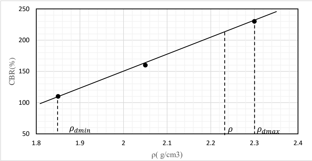
图E. 1 CBR 与干密度的关系
