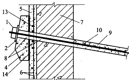
(b) 预应力锚杆、承压板与面层
