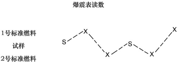
图5 试样和标准燃料读数顺序
