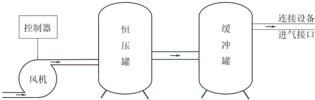
图2 进气增压恒压装置
