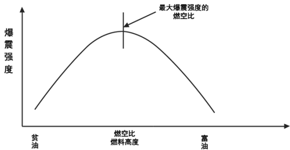
图4 燃空比对爆震强度的影响
