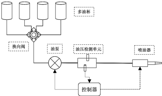
图3 燃油系统
