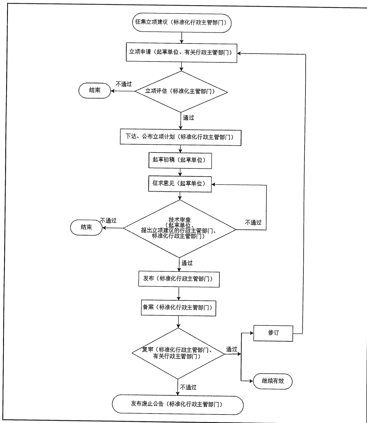
图A.1 地方标准制(修)订流程
