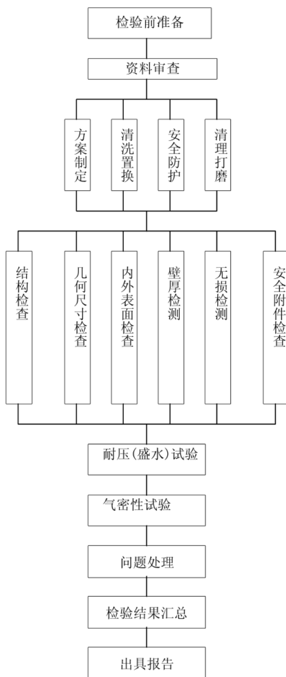
图 3 固定式常压储罐定期检验工作程序
