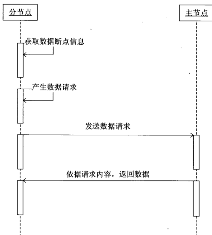
图 7 断点续传流程
