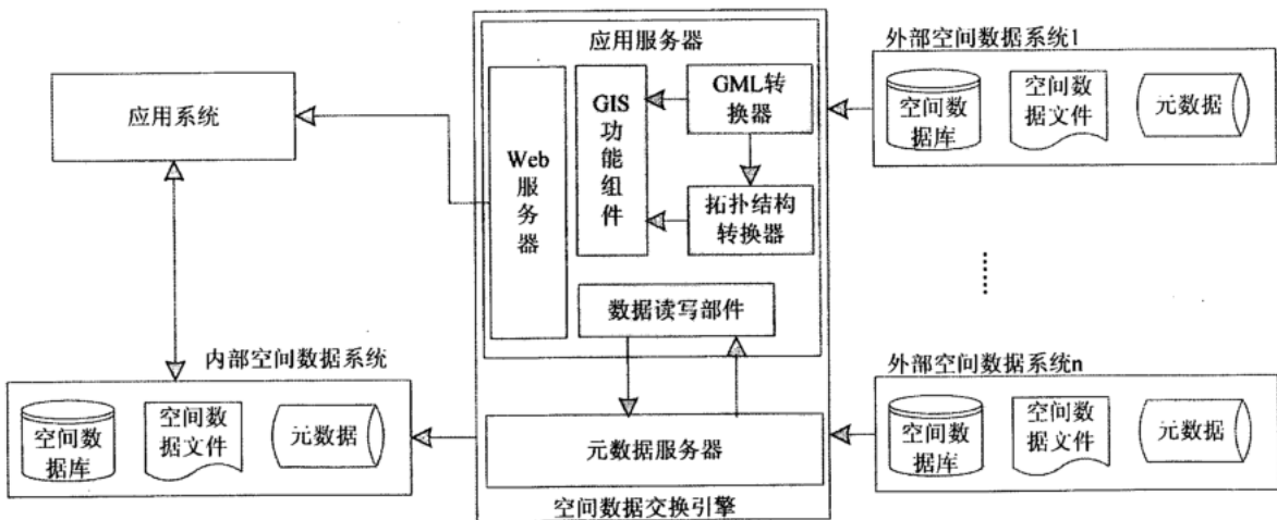
图 1 环境空间数据交换模型构成
