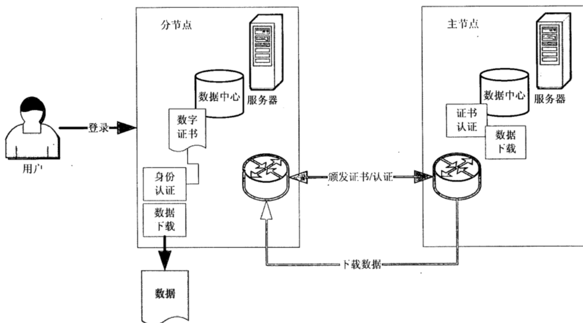
图5 数据下载流程
