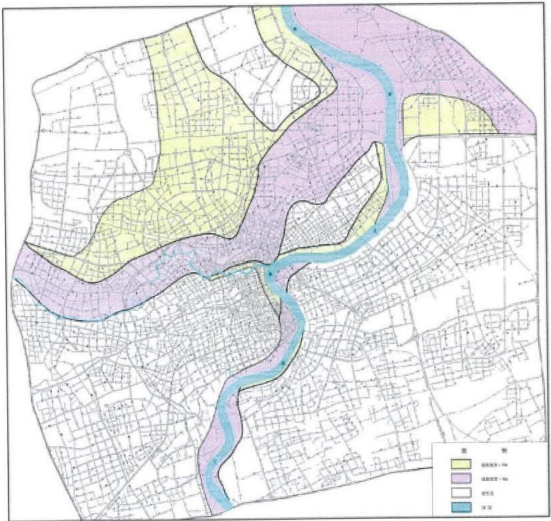
图 J.1 上海市区浅层粉性土和砂土层分布图
