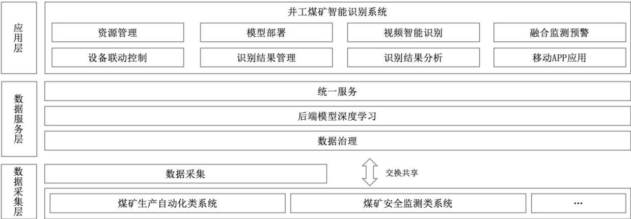
图 2 系统结构图
