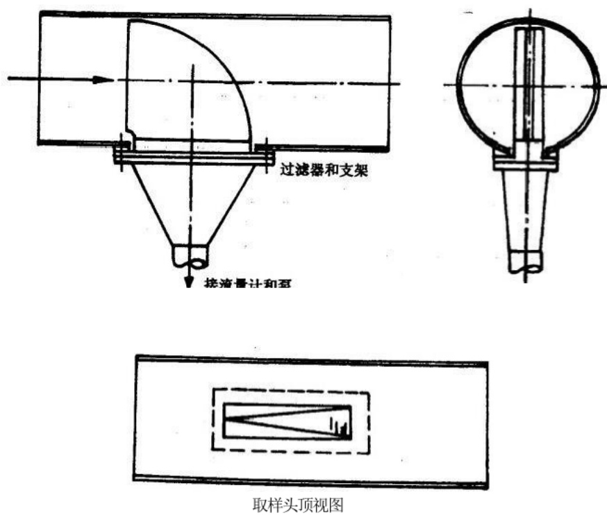
图 B3 单点取样的矩形缝状取样头人口及取样头
