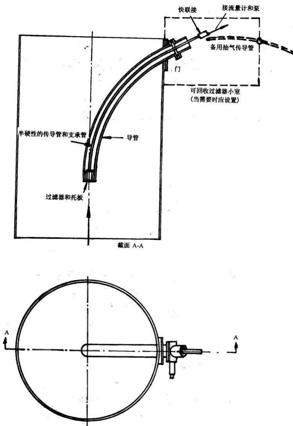
图 B4 无传导损失单点取样的取样头
