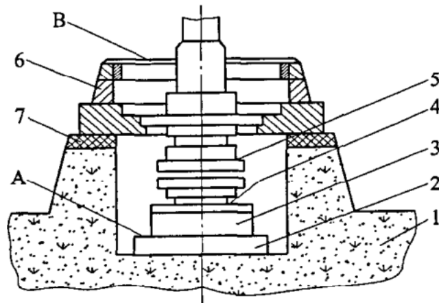
图 11.0.1 磨粉机安装
