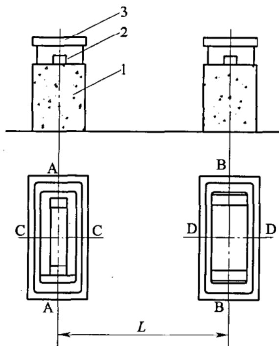
图 9.1.1 主轴承底盘组装
