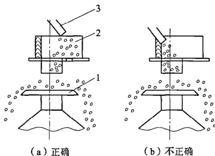
图 5.0.11 给料槽组装
