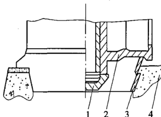
图 2.0.1 通道壁上预埋固定的金属护板
