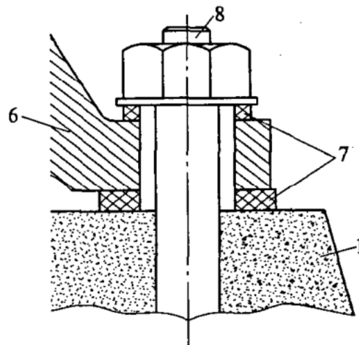
图 11.0.2 安装防震垫
