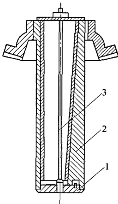
图 5.0.4-2 偏心套组装
