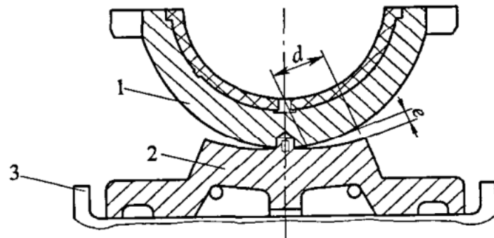
图 9.1.5 主轴承与轴承座的装配
