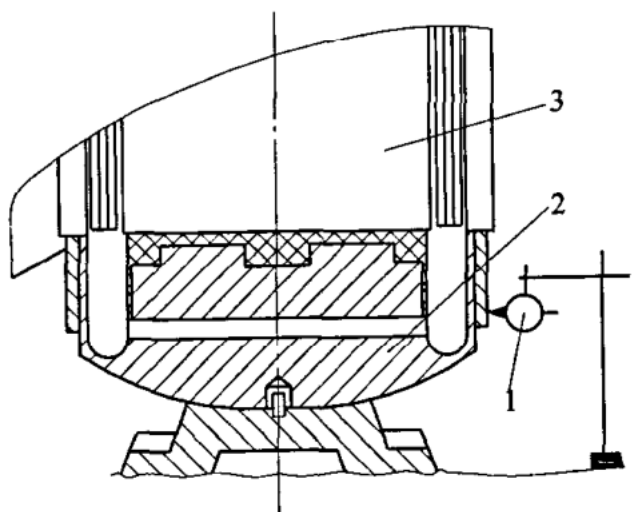
图 9.2.4 检查主轴承端面跳动
