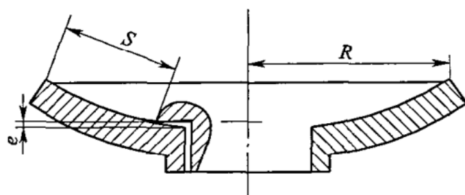
图 5.0.7 破碎圆锥与碗形轴承的配合
