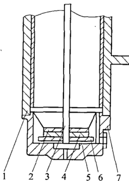
图 5.0.4-1 底托盘的调整垫片和止推垫组装
