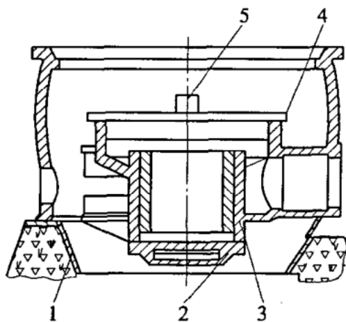
图 4.0.1 机座的安装水平检验
